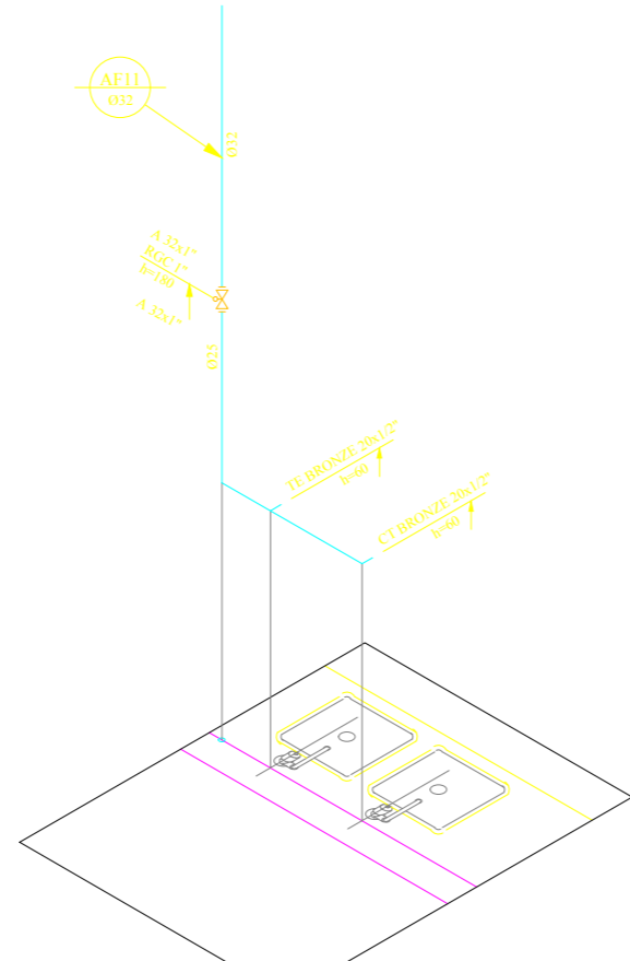
DET. A9
