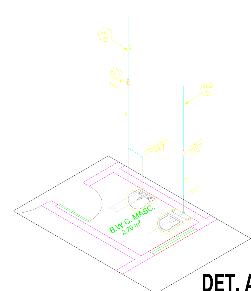
DET. A7
