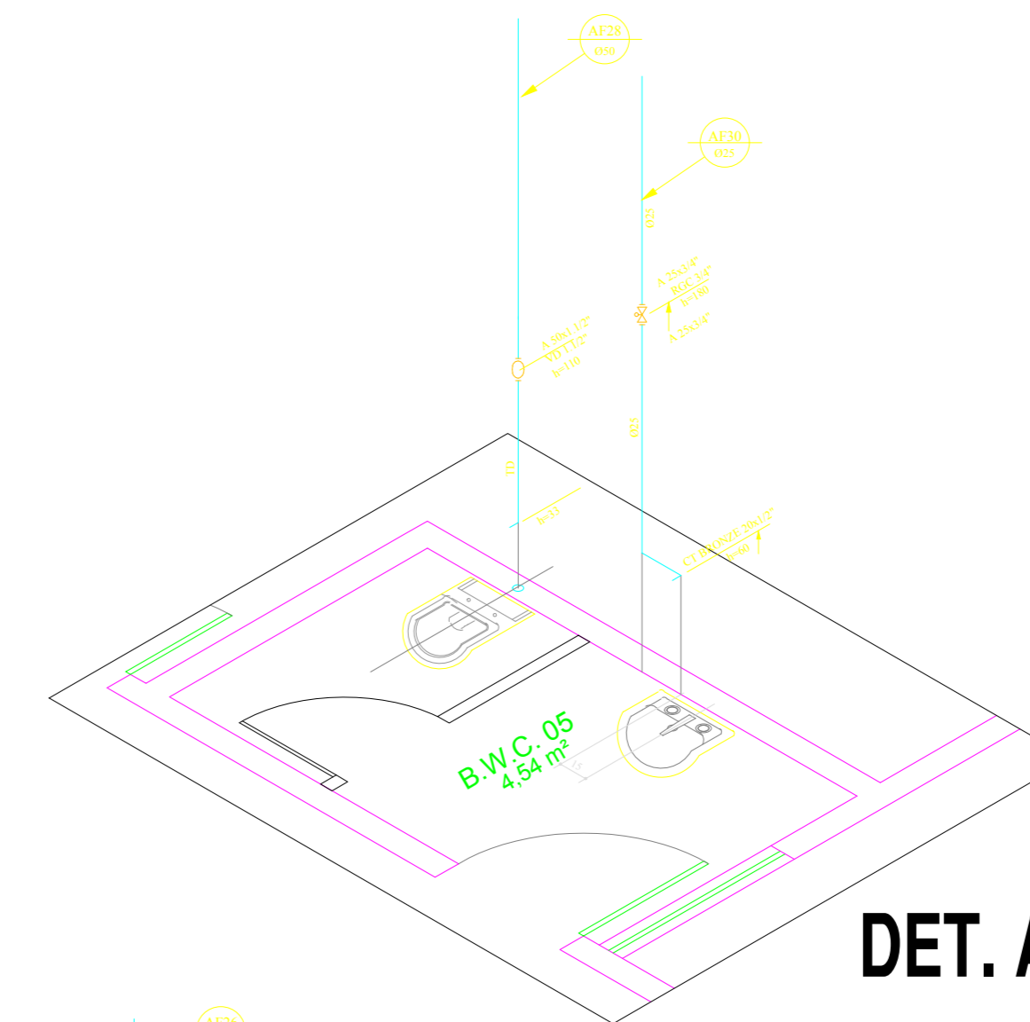
DET. A14
